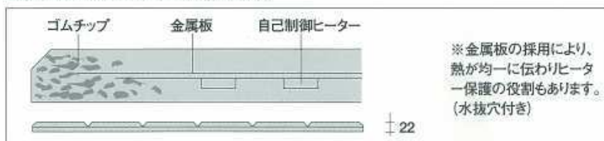
電気融雪パネル「Gマット」断面図
